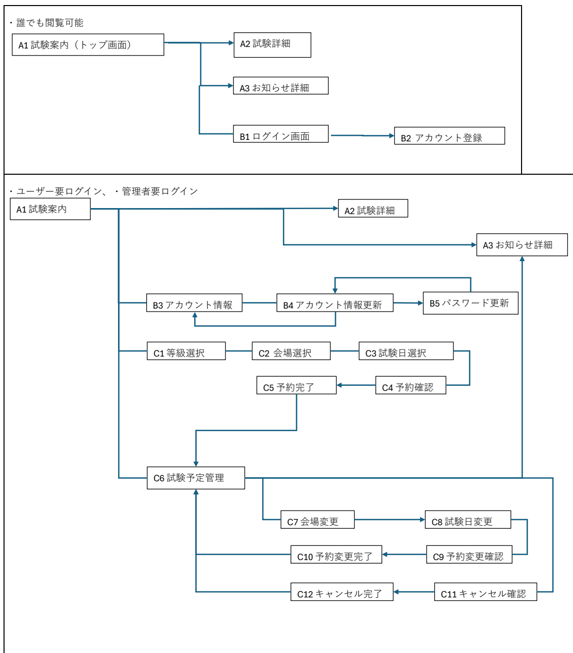
画面遷移図
